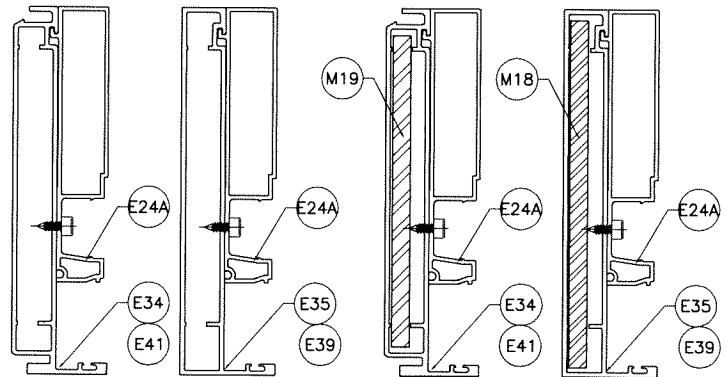
JAMB 'J1A'
